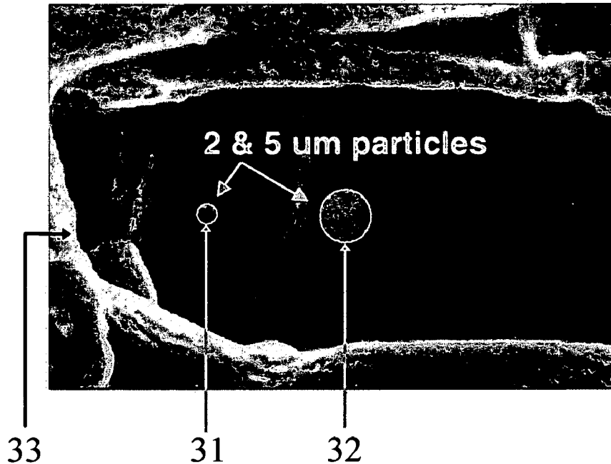
FIG. 3A Cellulose Media
